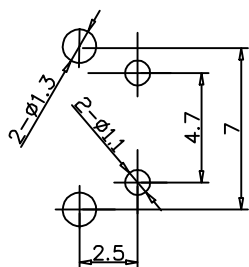
安装孔位图
